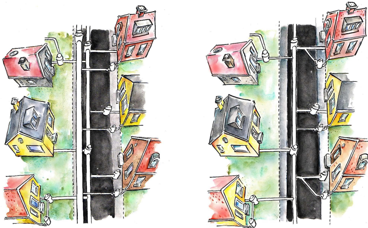
Separatsystem: Spildevand og regnvand i rør hver for sig Fællessystem: Spildevand og regnvand i samme rør
